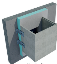
Illustration pour l'isolation périphérique avec 2 paires d'équerres de fixation
